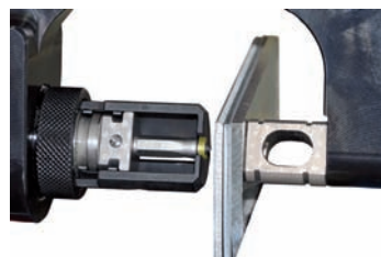
Punzonador para la realización de orificios, incluso en aceros de ultra alta resistencia.
